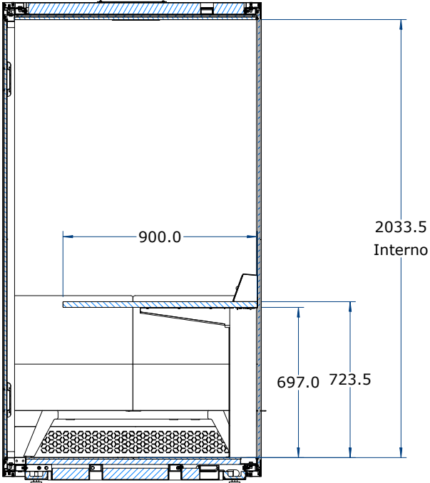
SECCIÓN C-C ESCALA 1 : 25
