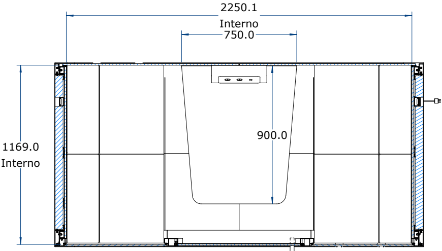
SECCIÓN D-D ESCALA 1 : 25
