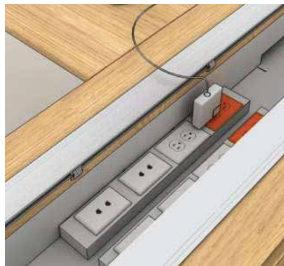
Conexión superior
